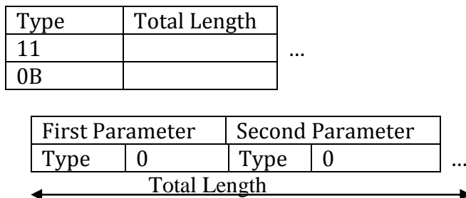
Figure 3-4 Get Parameter TLV example
