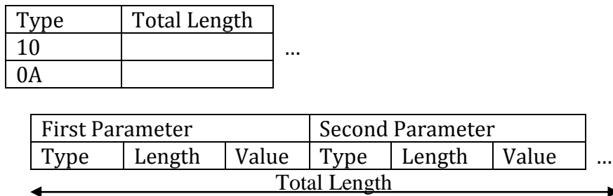
Figure 3-3 Set Parameter TLV example
